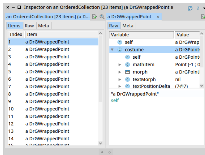
Figure 9.7: L'inspecteur sur la variable sommets
