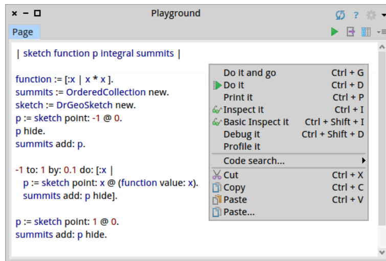
Figure 9.1: Votre espace de travail avec le code source collé et son menu contextuel
