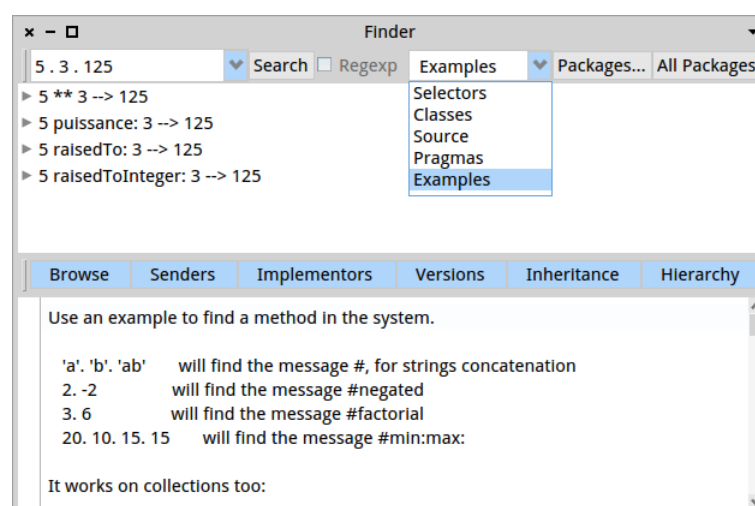
Figure 9.10: Réponse du Chercheur sur un motif de calcul et sa réponse souhaitée
