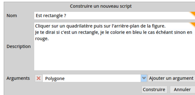
Figure 6.4: Le constructeur de script avec un argument demandé
