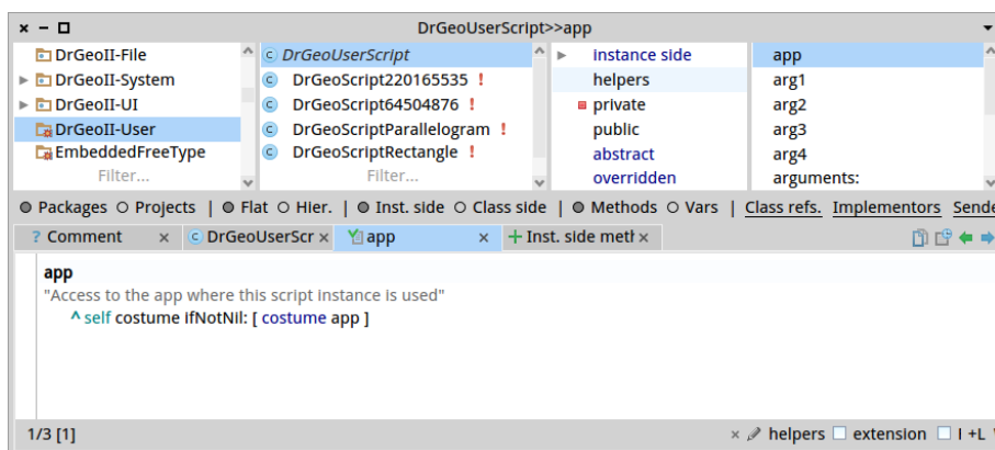
Figure 6.6: Navigateur de classe Calypso
