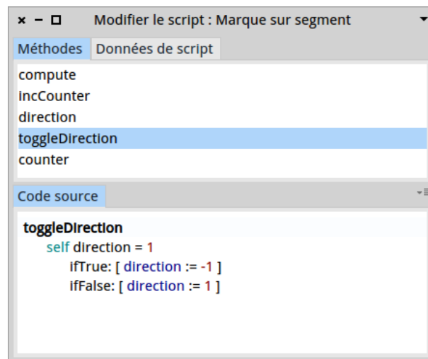
Figure 1.9: Éditer un script
