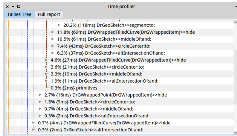
Figure 9.5: Le profileur Dr.Geo à l'issue de la construction de la courbe de Sierpinski
