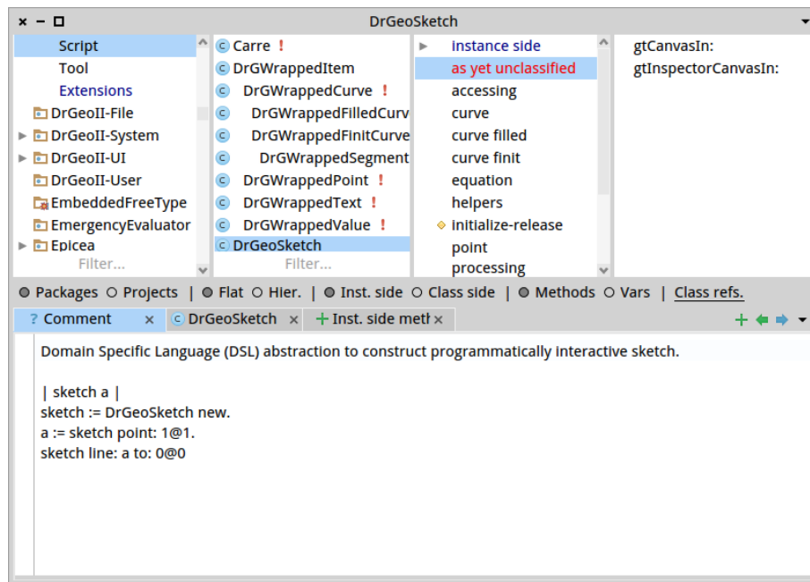
Figure 2: La navigateur du code source de Dr.Geo depuis Dr.Geo lui-même
