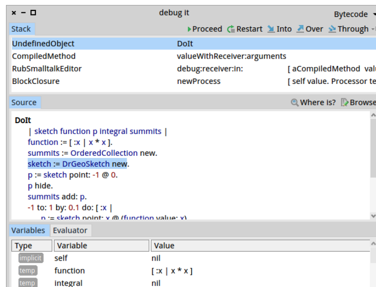
Figure 9.6: Le débogueur Dr.Geo
