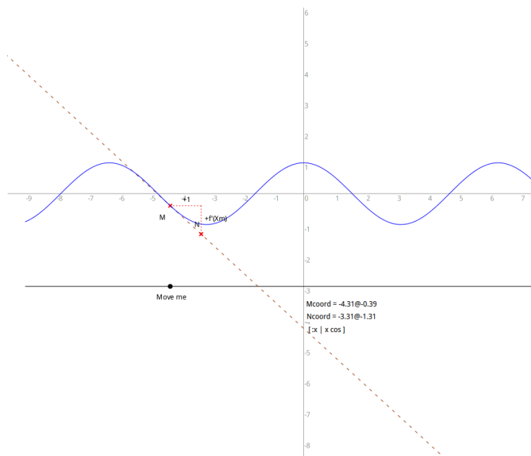
Figure 6.5: Courbe et tangente en un point
