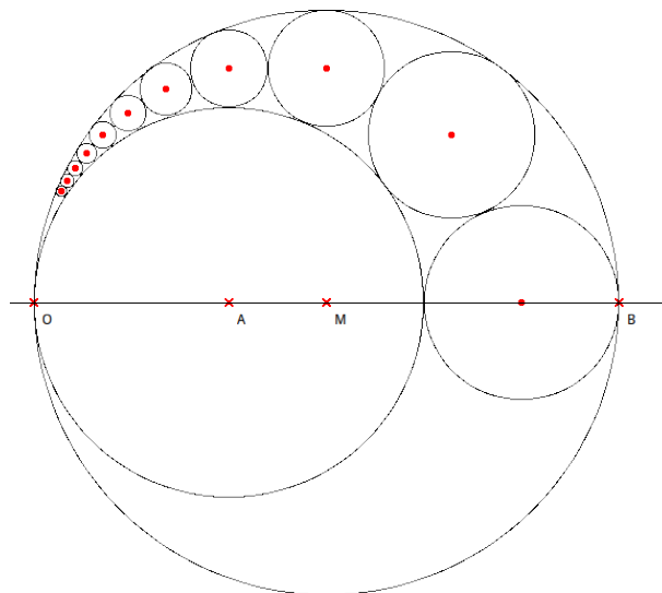
Figure 8.11: Catena di Pappo
