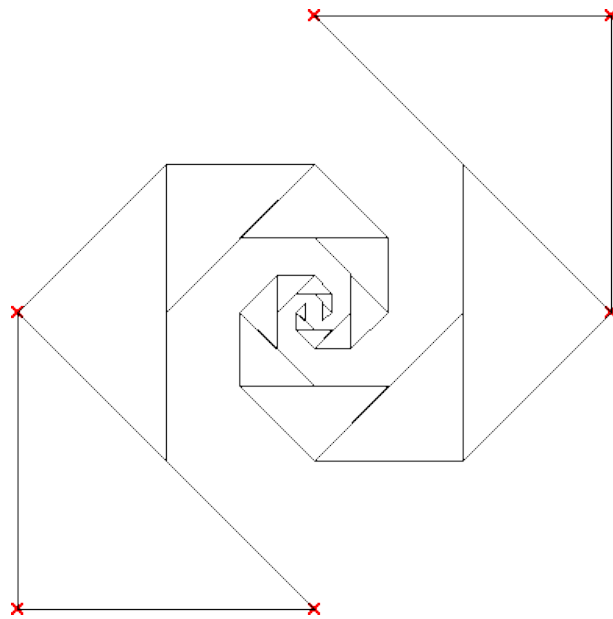
Figure 8.10: La spirale de Baravelle suite à l'exécution du code Pharo
