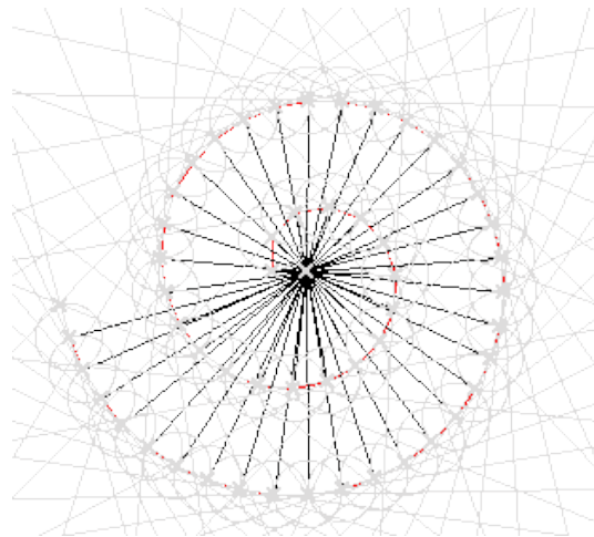
Figure 8.9: Spirale de Teodoro avec les éléments cachés révélés
